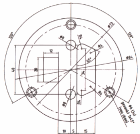
Maßbild Sockel
