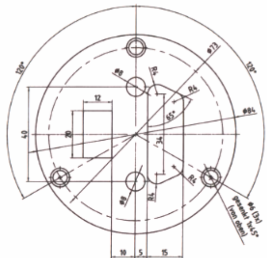
Maßbild Sockel
